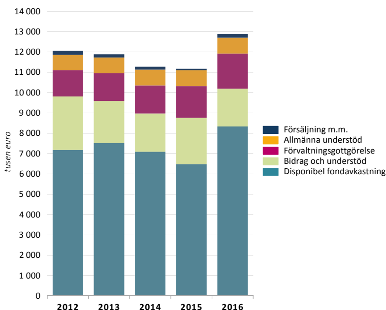
SLS intäkter
